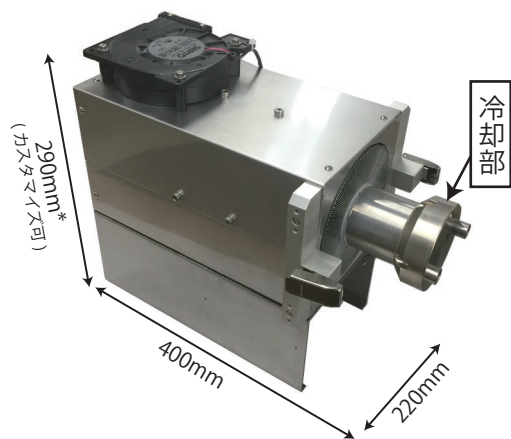
冷却装置本体
